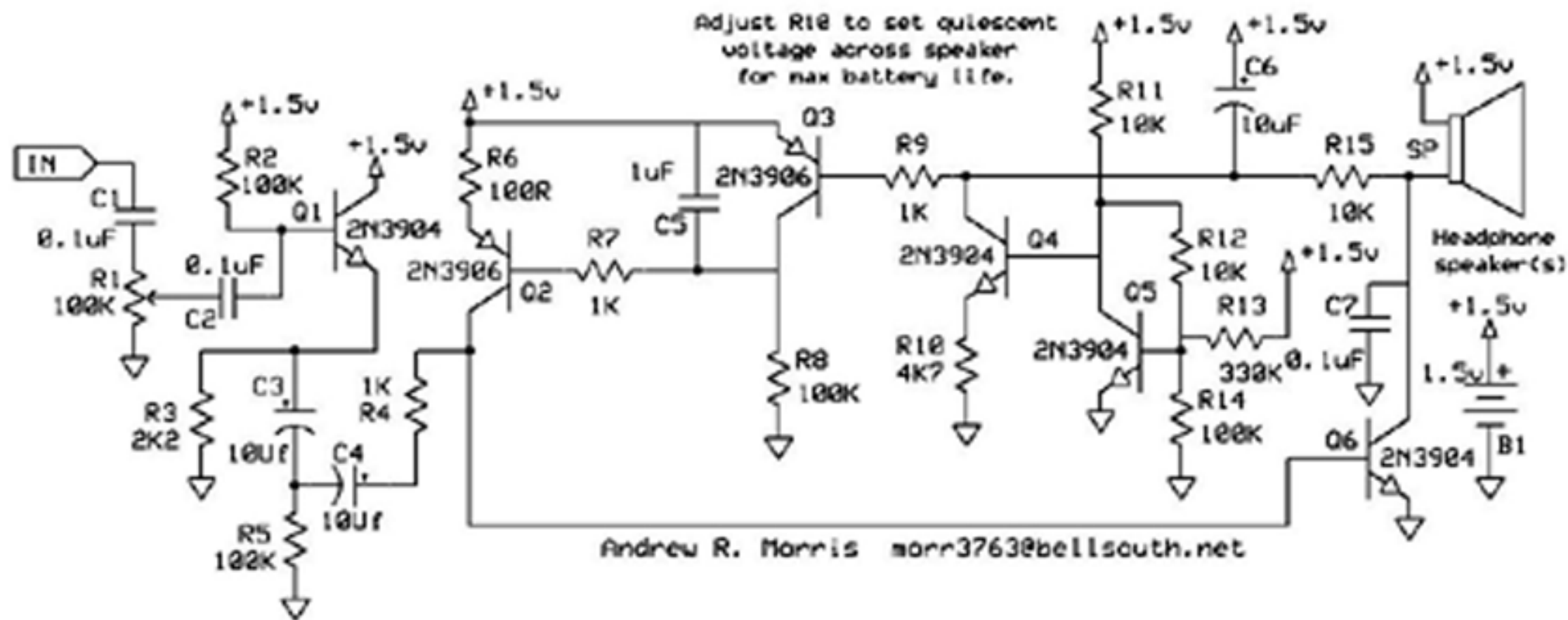
1.5 volt headphone amplifier
